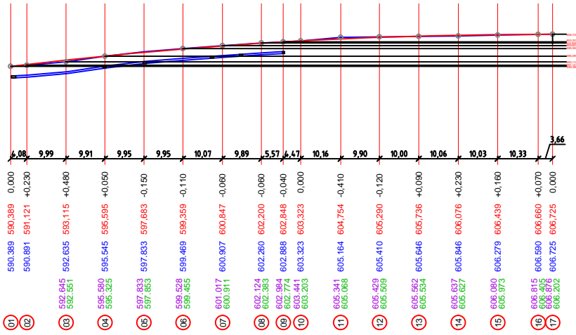
PERFIL LONGITUDINAL - TRAVESSA DOS SABIÁIS
